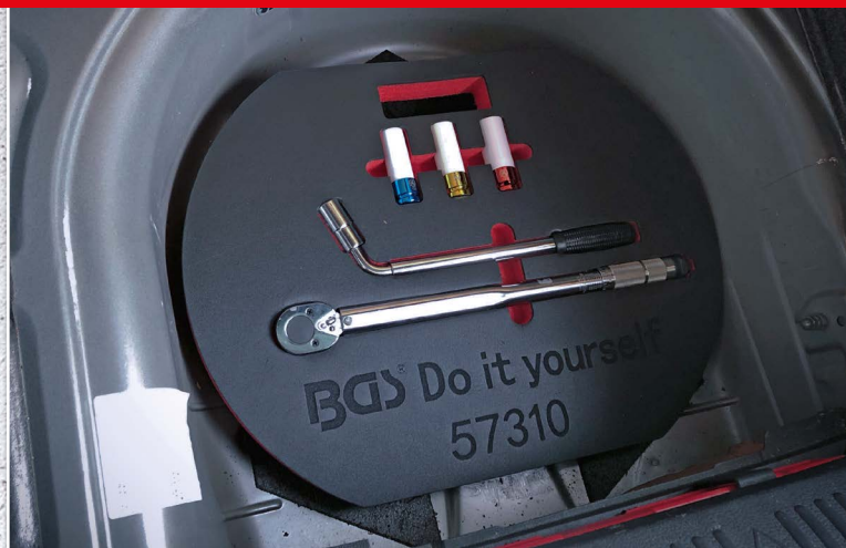
Radwechsel-Service-Satz | 5-tlg.
