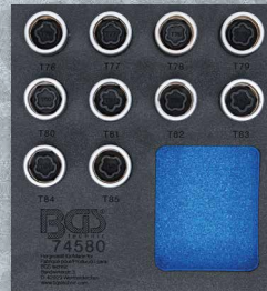
Werkstattwageneinlage 1/6: Felgenschloss-Werkzeug- Satz für Tesla | 10-tlg.
